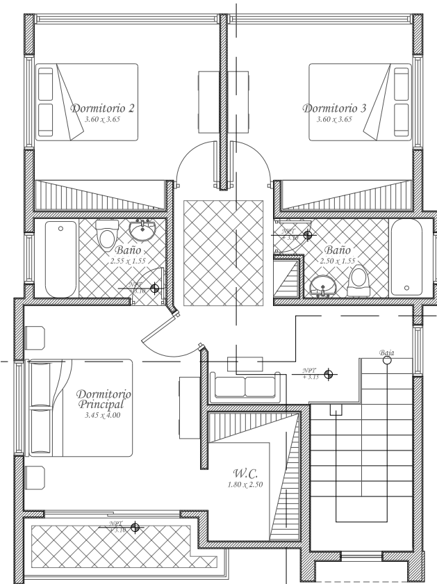
SEGUNDA PLANTA
